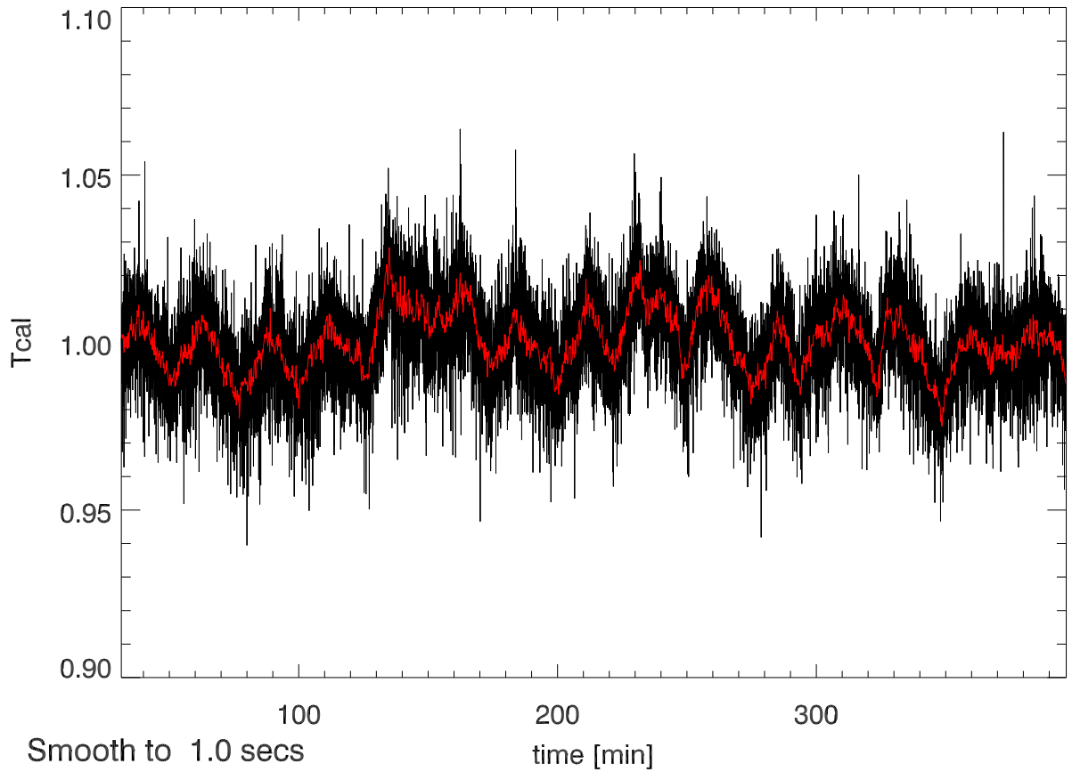
05jun12 calOn - calOff Beam0A SigA: 0.019
