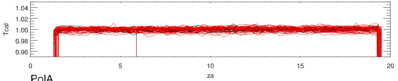
30apr11 a2130 alfaCalDeflection vs za beam0
