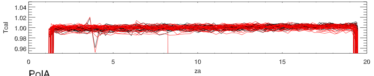
23jun11 a2130 alfaCalDeflection vs za beam0
