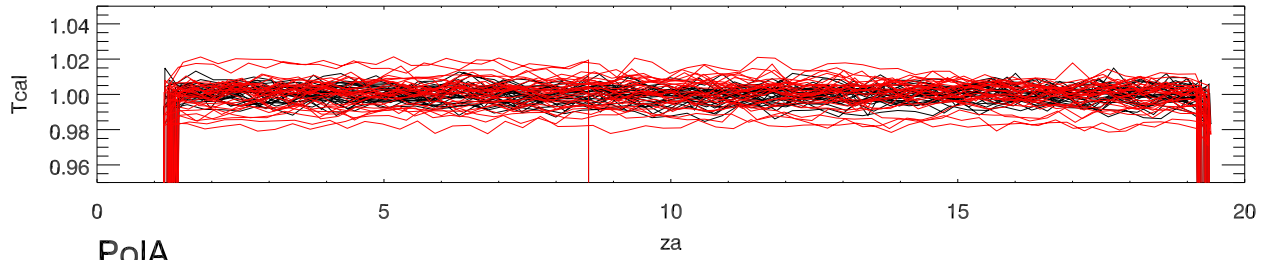
20oct11 a2130 alfaCalDeflection vs za beam0
