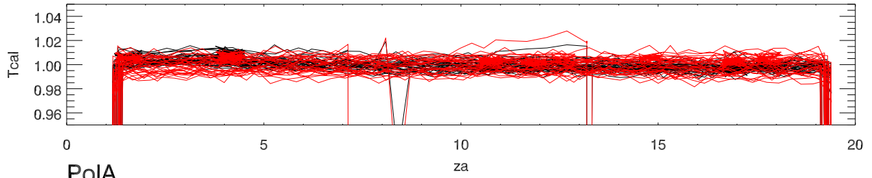
07nov11 a2130 alfaCalDeflection vs za beam0
