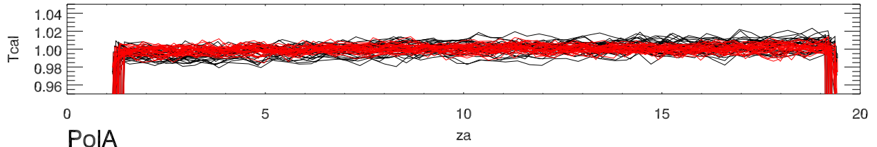
03may12 a2130 alfaCalDeflection vs za beam0
