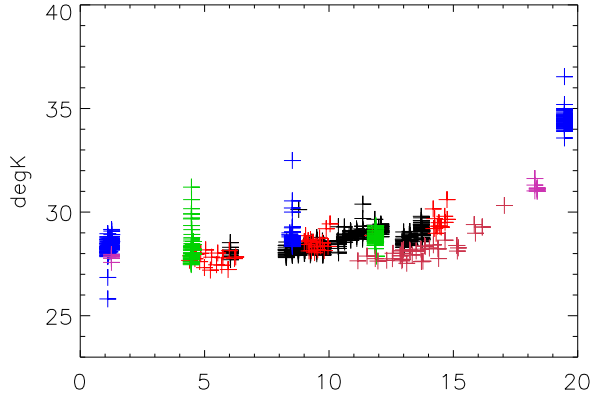
dec06 Alfa Tsys vs za Pixel 0 Pol A
