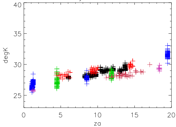
dec06 Alfa Tsys vs za Pixel 2 Pol A
