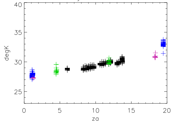
dec06 Alfa Tsys vs za Pixel 2 Pol B
