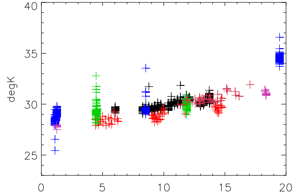
dec06 Alfa Tsys vs za Pixel 0 Pol B
