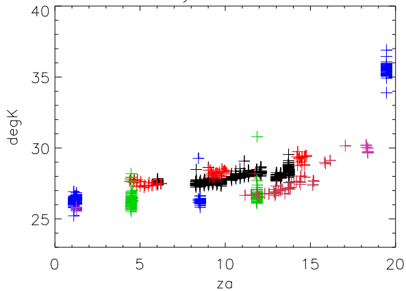
dec06 Alfa Tsys vs za Pixel 3 Pol A
