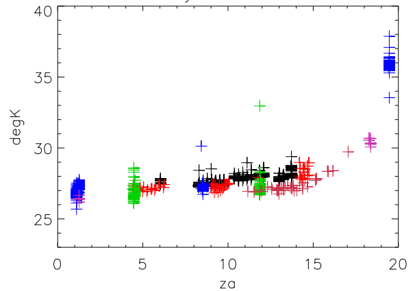
dec06 Alfa Tsys vs za Pixel 3 Pol B
