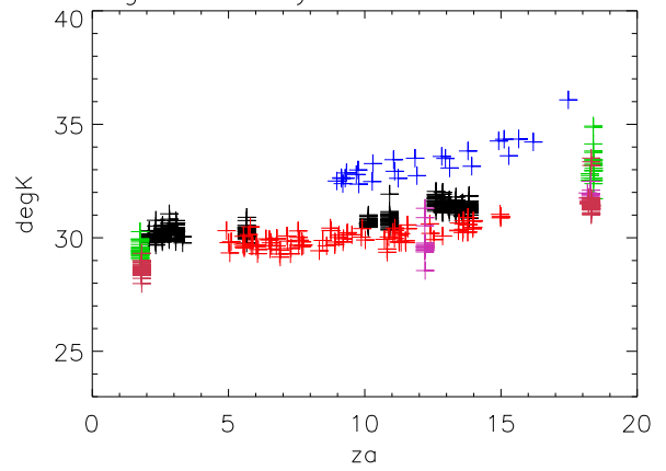
aug06 Alfa Tsys vs za Pixel 1 Pol B
