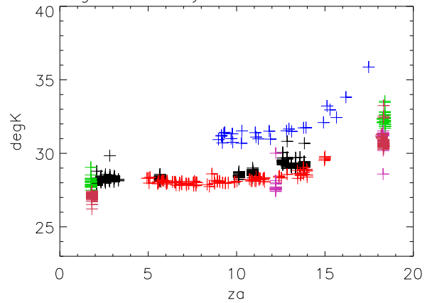
aug06 Alfa Tsys vs za Pixel 3 Pol B
