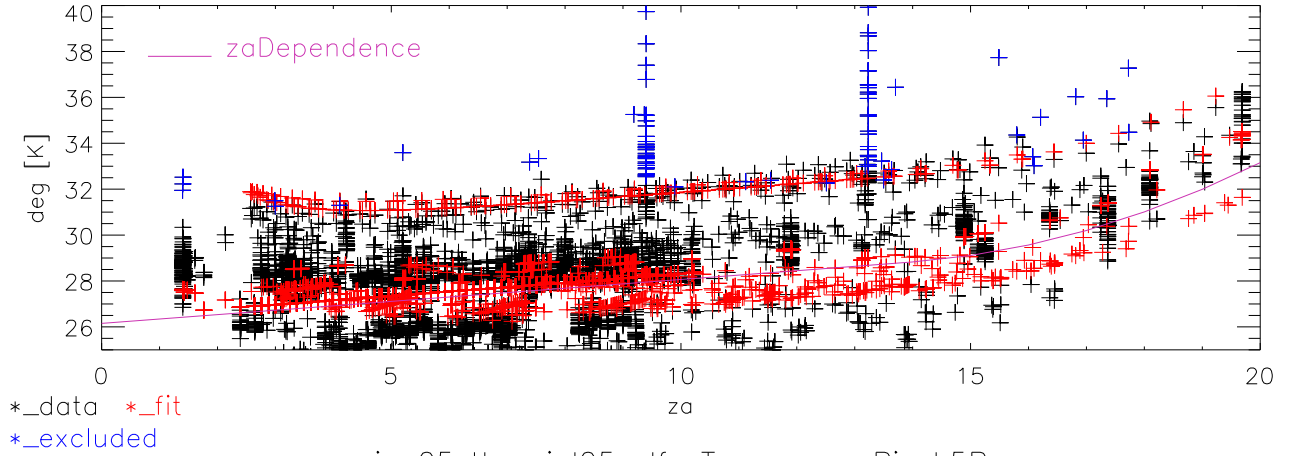
jan05 thru jul05 alfa Tsys vs az Pixel:5B
