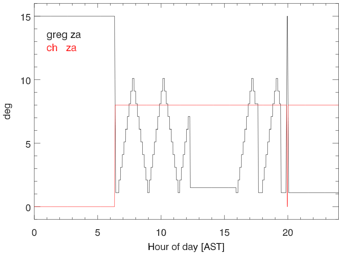
00161106 za Position vs hr
