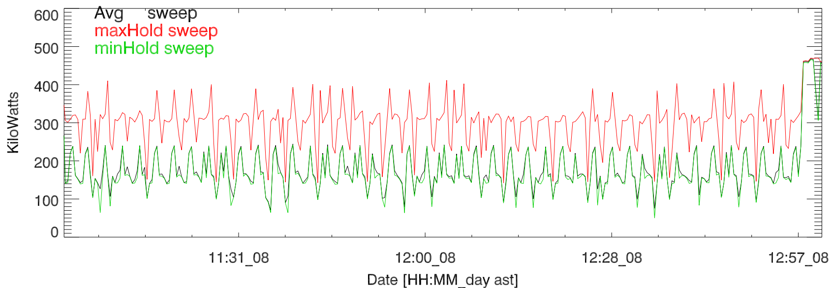
TxPwrTot. 08nov18:H3251 5 MHz
