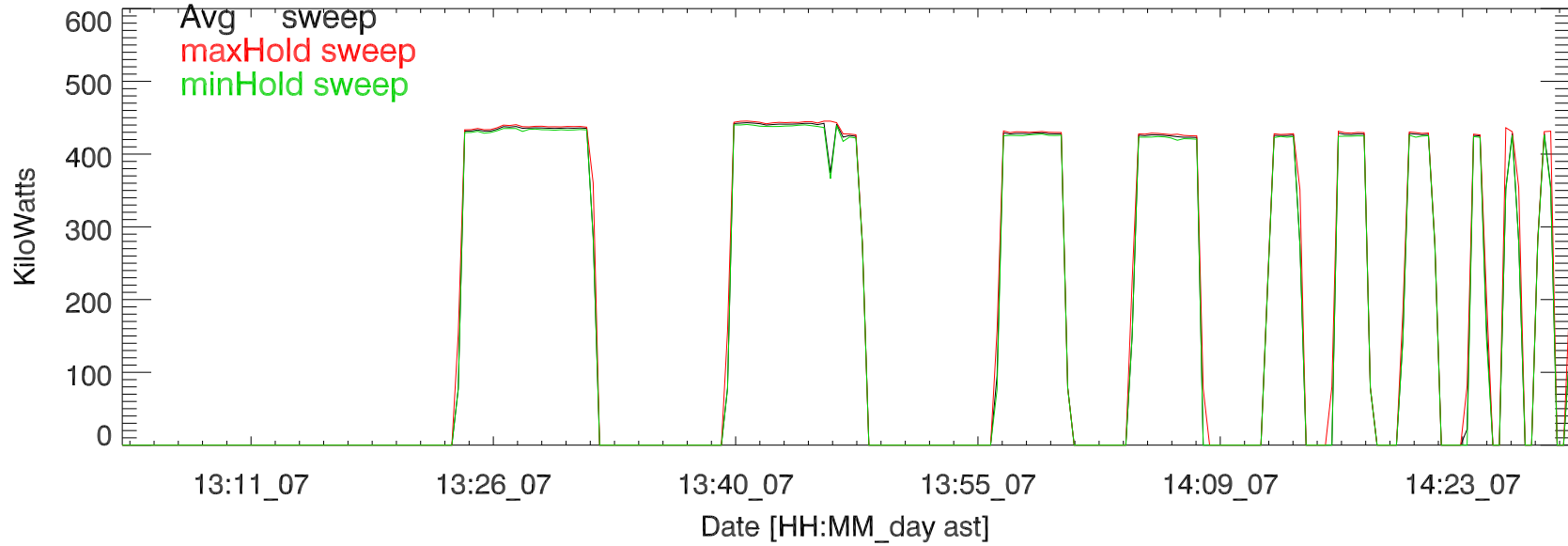
TxPwrTot. 07nov18:H3211 5 MHz
