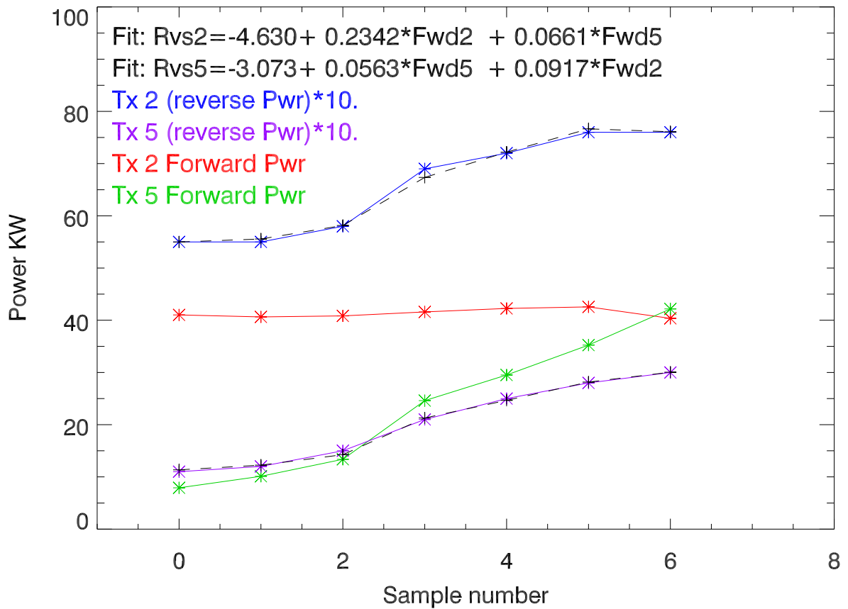
Tx2,5 Fit RvsPwrTx2= a_0 + a_1 \cdot \text{fwdTx2} + a_2 \cdot \text{fwdTx5}
