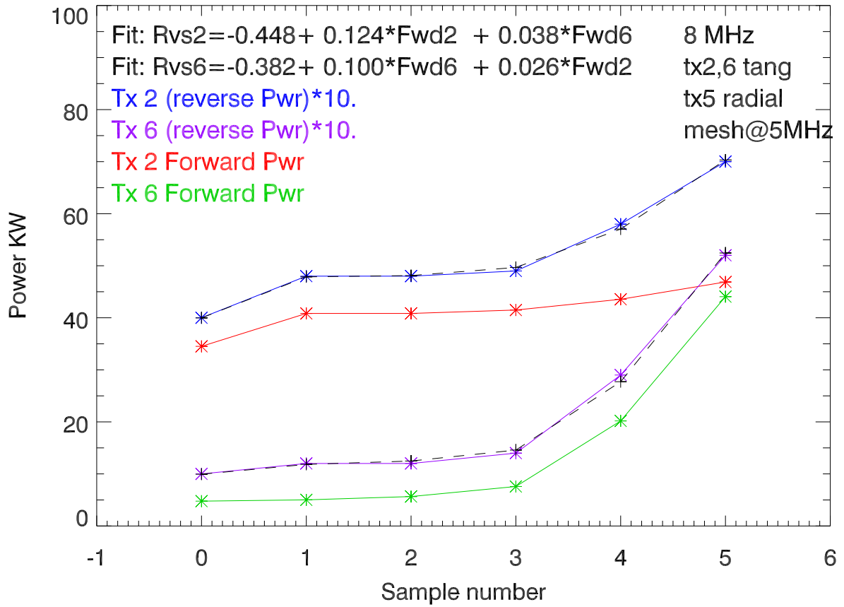
Tx2,6 Fit RvsPwrTx2= a_0 + a_1 \cdot \text{fwdTx2} + a_2 \cdot \text{fwdTx6}
