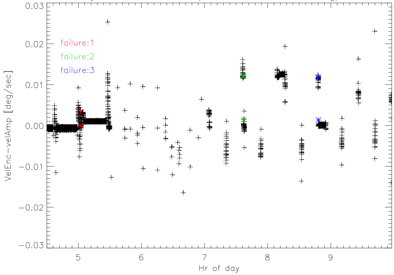
31jan10 velEnc-velAmp when velEnc < .01 deg/sec
