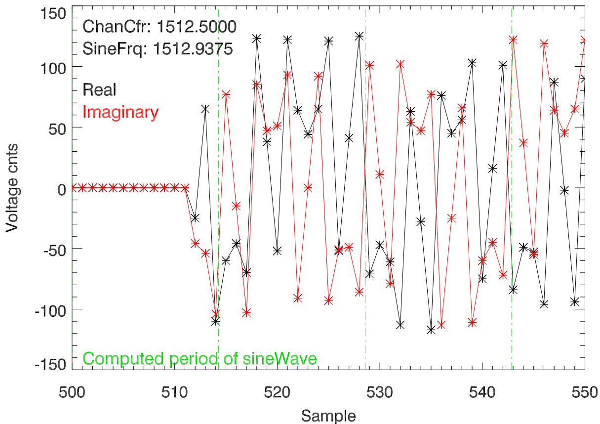
chan14 (gpu05,ch 2) Voltage vs sample. SineWaveChan
