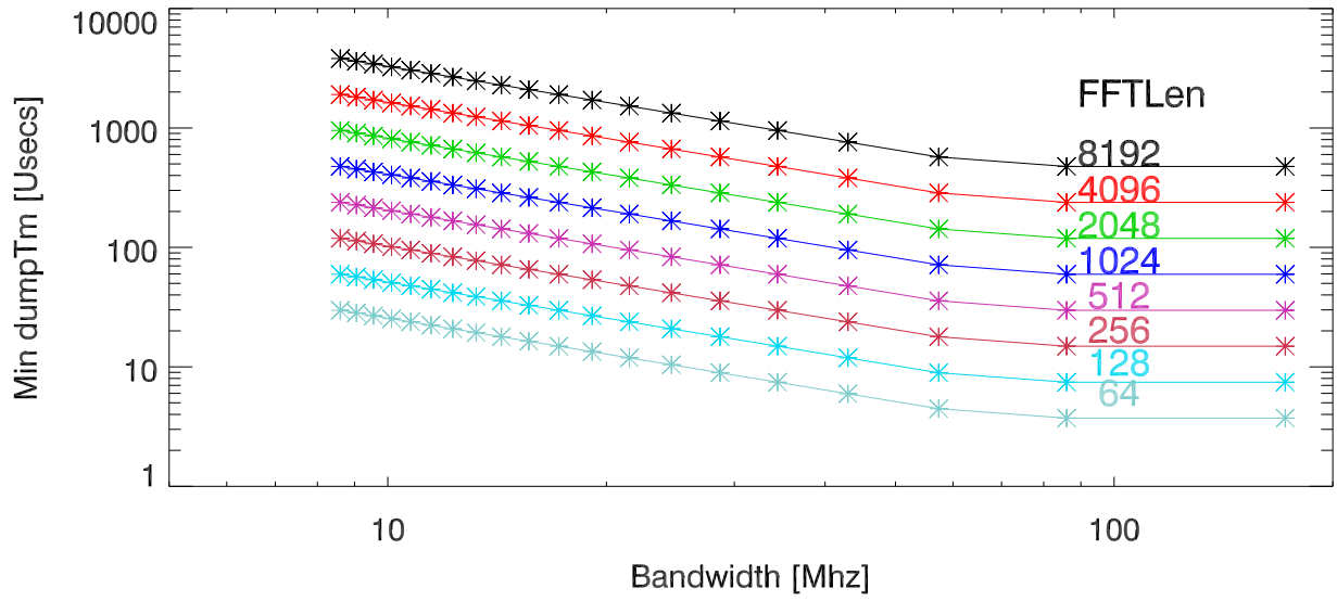
Mock Min dump times. ALFA. (Sum PoIS)
