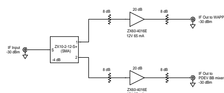
ALFA / WAPP IF Splitter
