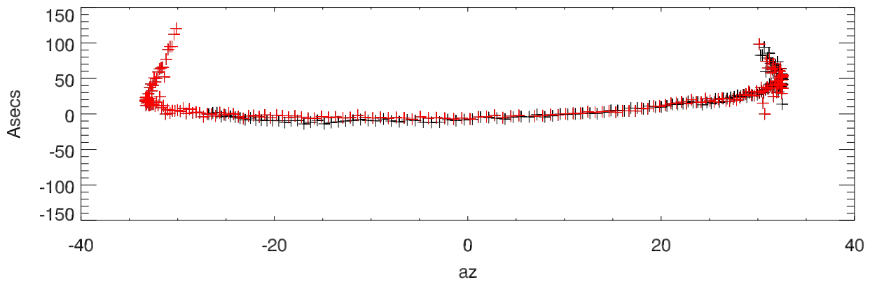
3C461 El pointing errors vs az
