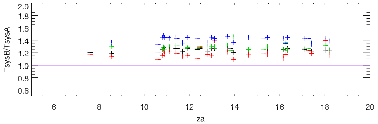
TsysPoIB/TsysPoIA Vs Za
