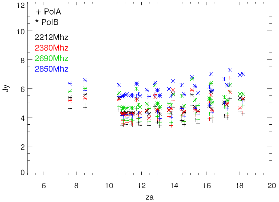
SEFD Vs Za
