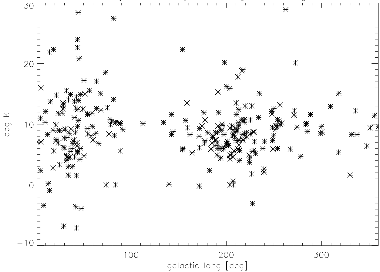
327 TsysPolB - TsysPolA vs galactic longitude
