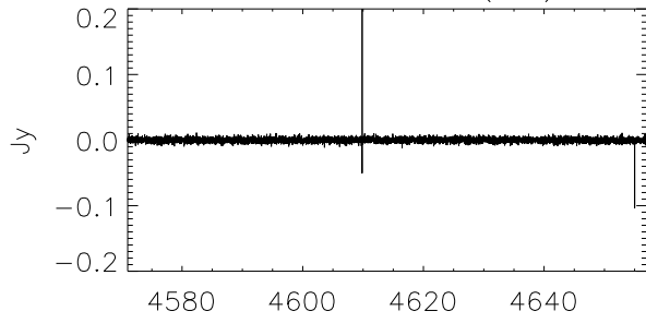
G188.95+0.89 (WB)
