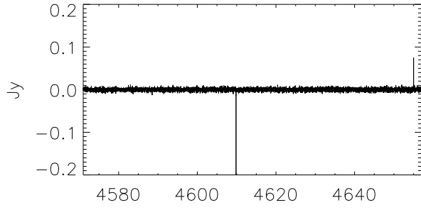
G206.05-2.57 (WB)
