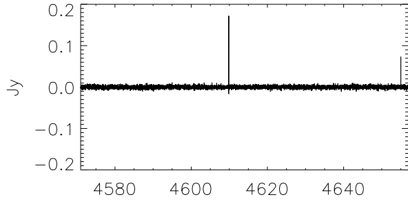
G188.90+0.76 (WB)
