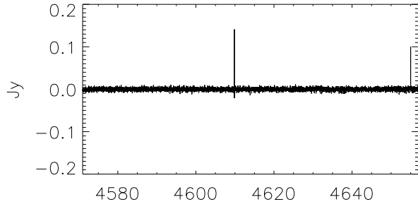
G206.84-2.37 (WB)
