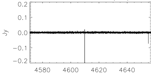
G188.95+0.88 (WB)
