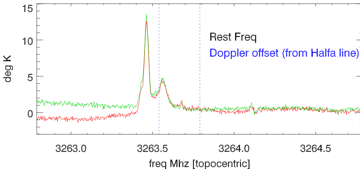
01jun10 a2463 SBH CH lines: 3263.79 Mhz
