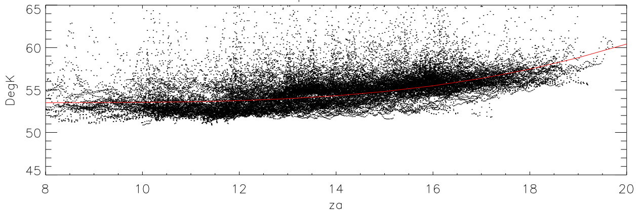
PolA data Epoch 2 data and fit.
