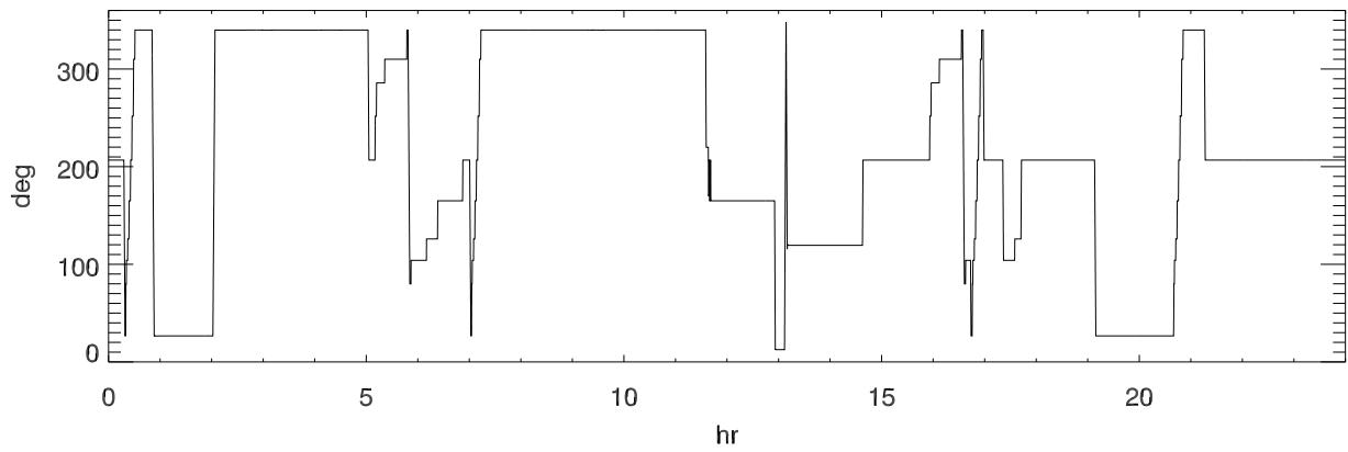
150601 turret Actual position
