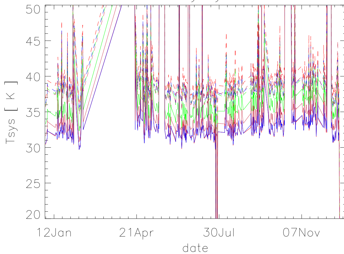
XBAND Tsys yr:2016
