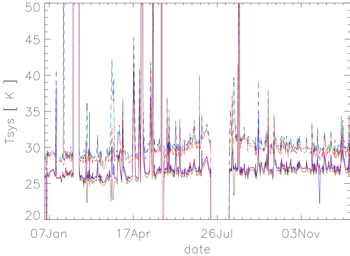
CBAND Tsys yr:2013
