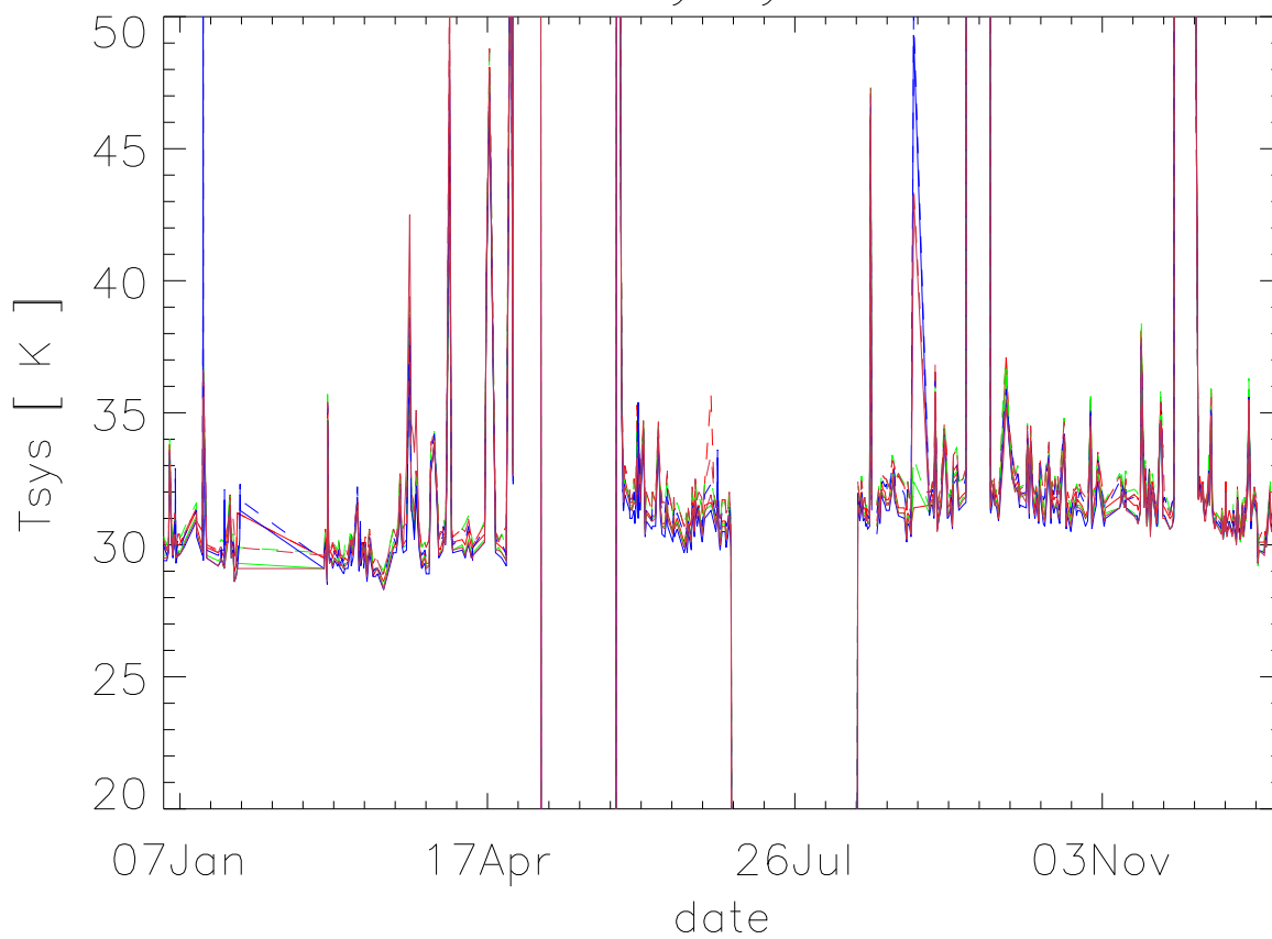
CBH Tsys yr:2013
