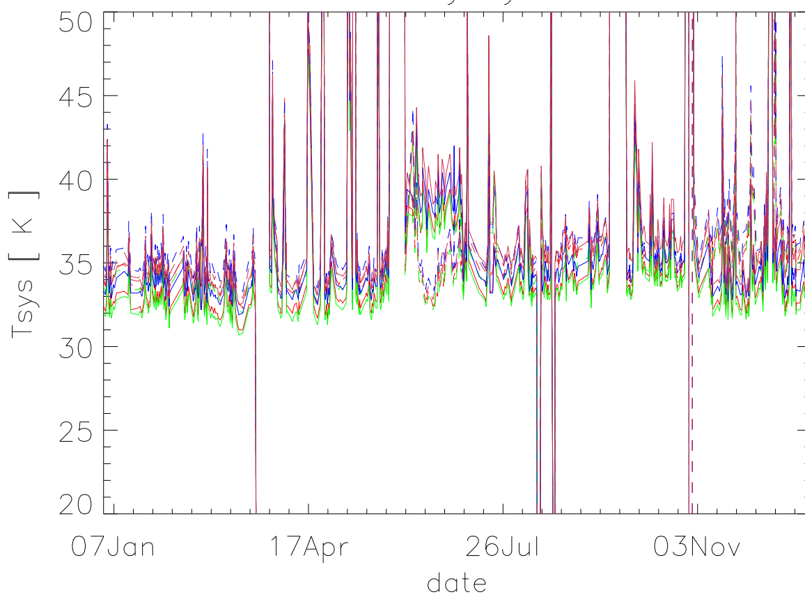
XBAND Tsys yr:2013
