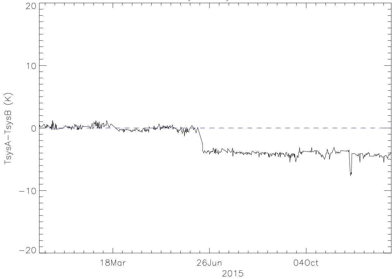
cbh TsysA-TsysB 2015
