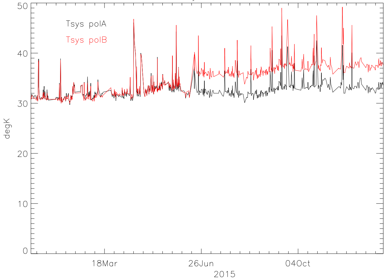
cbh TsysA-TsysB 2015
