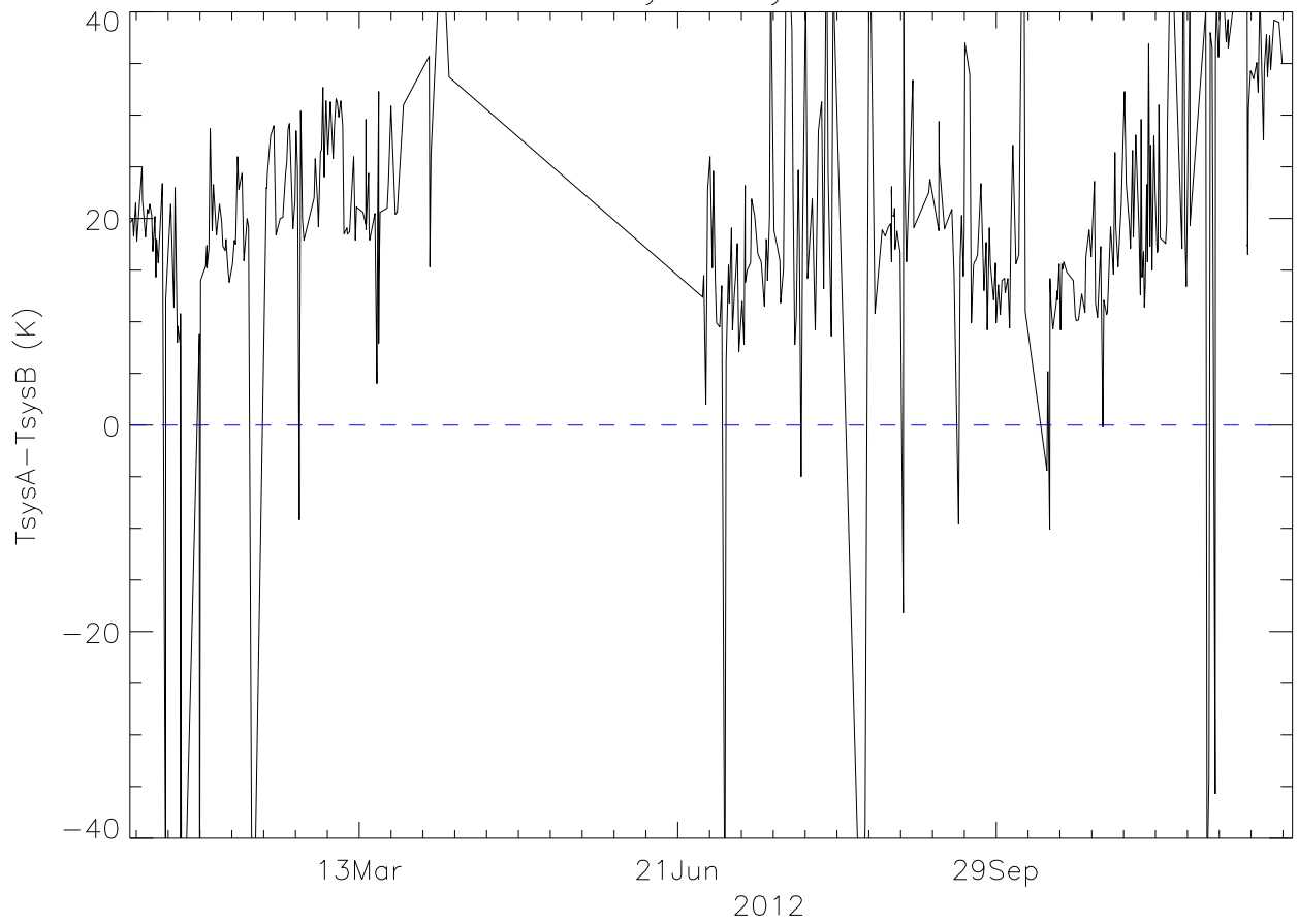
430ch TsysA-TsysB 2012
