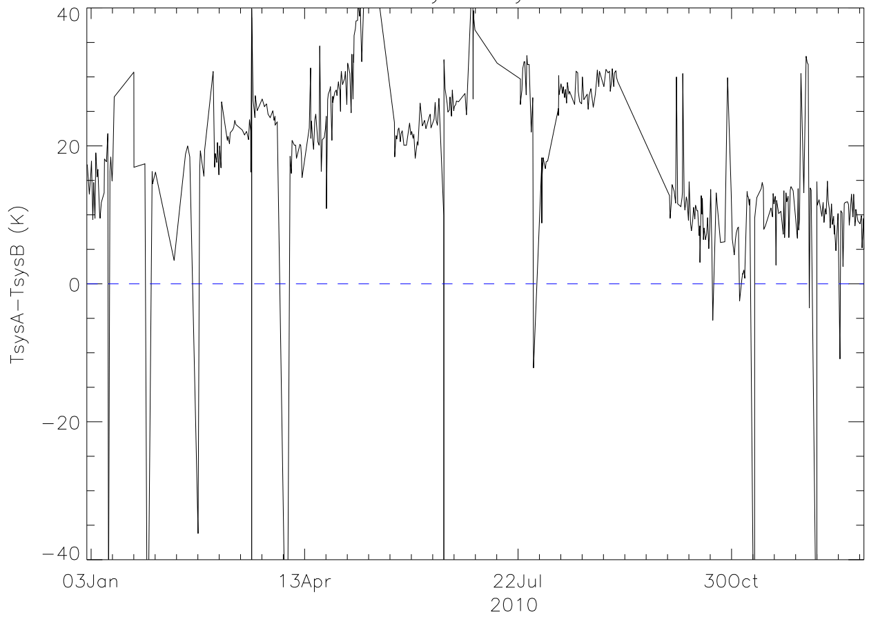
430ch TsysA-TsysB 2010
