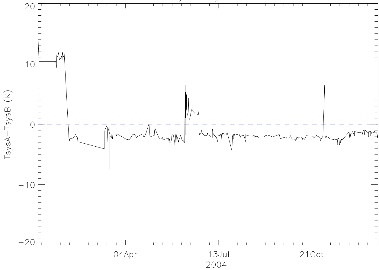
xb TsysA-TsysB 2004
