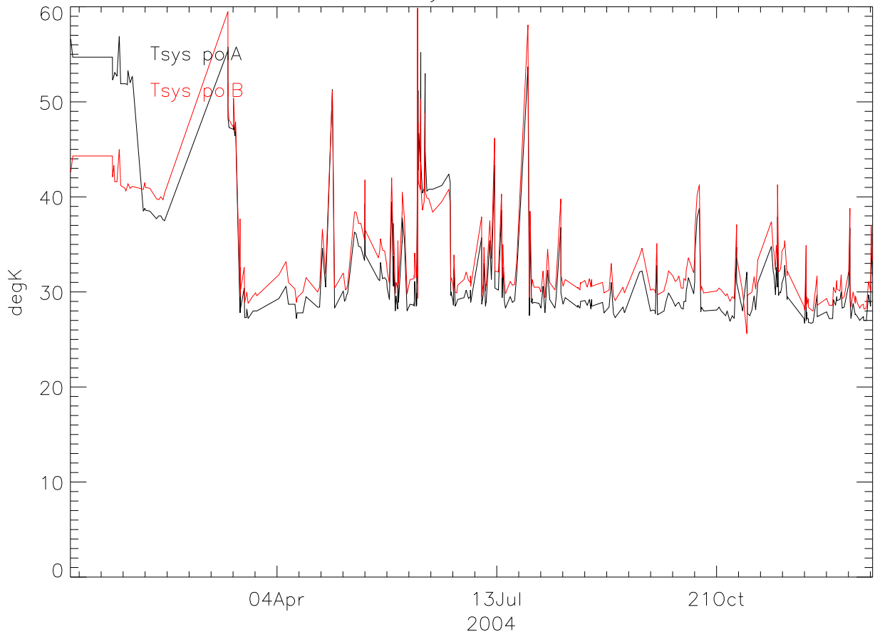
xb TsysA-TsysB 2004
