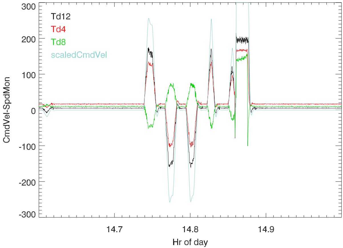
10feb12 CmdVel -spdMon. SignalCond R1=22K ohms
