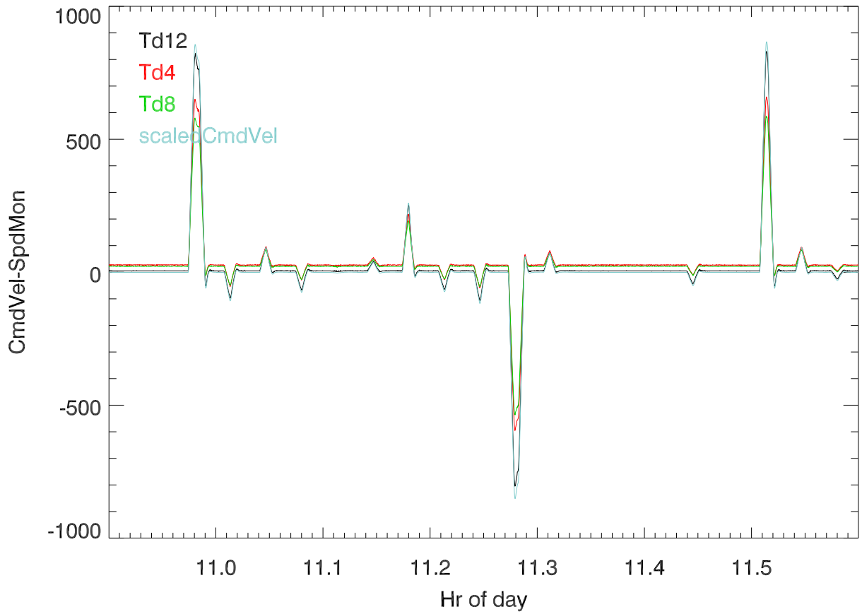
11mar11 CmdVel -spdMon. SignalCond R1=46.2K ohms
