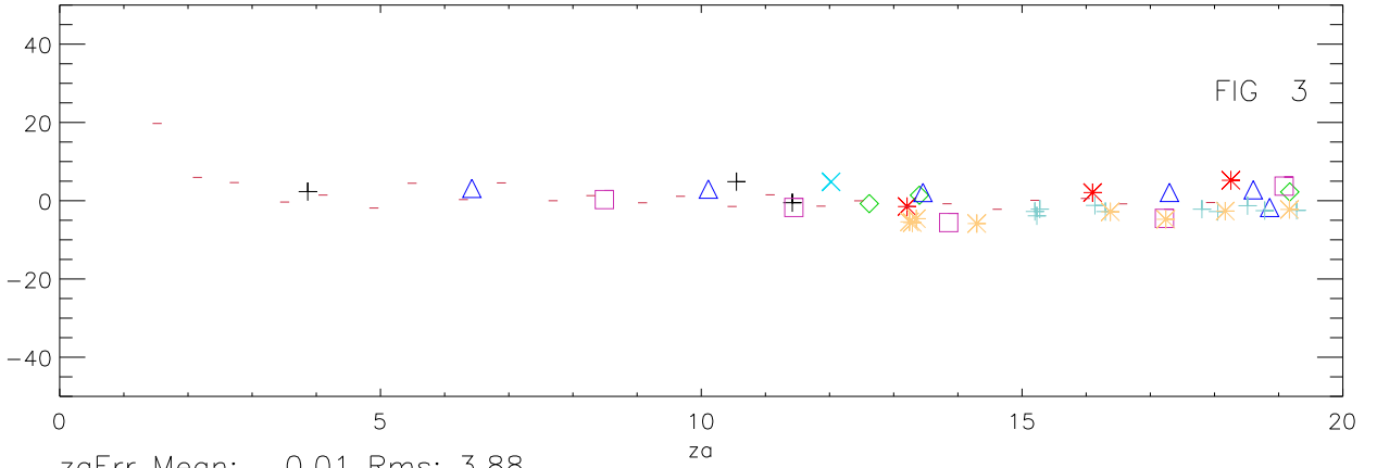
01apr12 to 30apr12 pixel 0 alfa 63 pnts. za error vs za
