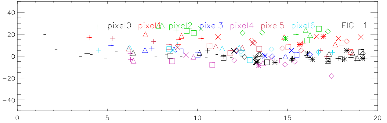
01apr12 to 30apr12 all Pixels alfa 158 pnts. za error vs za
