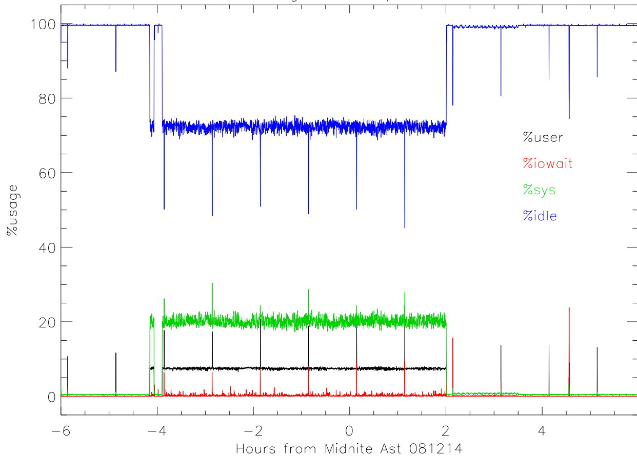
iostat CPU avg 10 secs.pdevs5 081214
