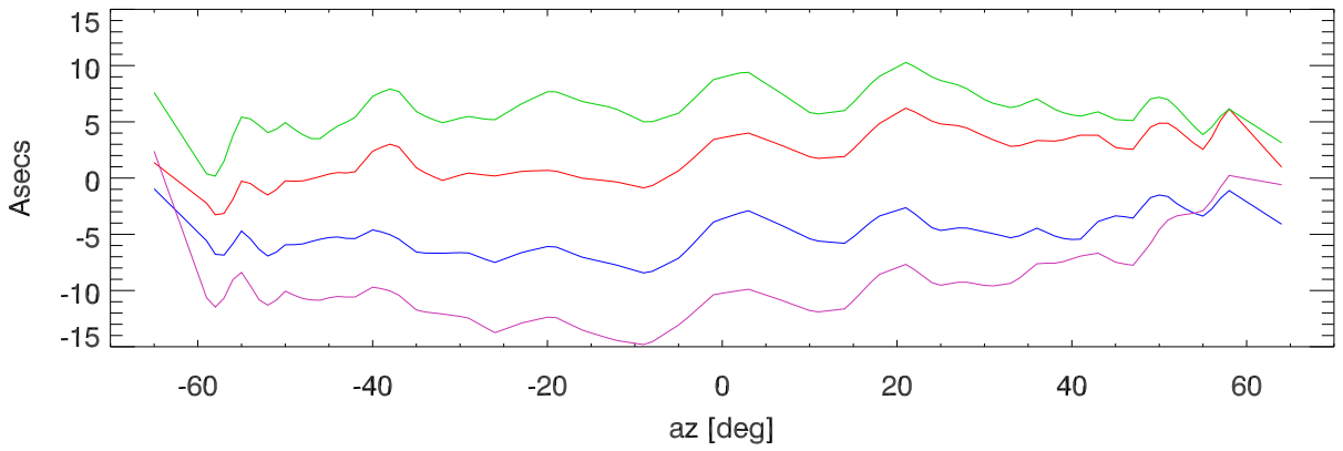
Za Errors vs az
