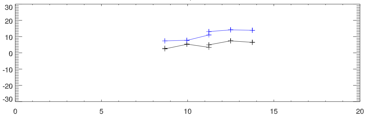
B2249+185 az,za error vs za
