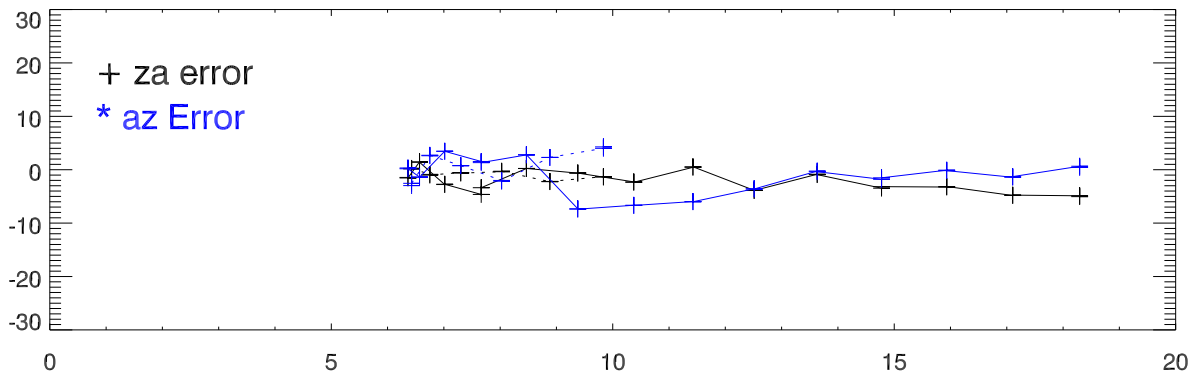
B1040+123 az,za error vs za
