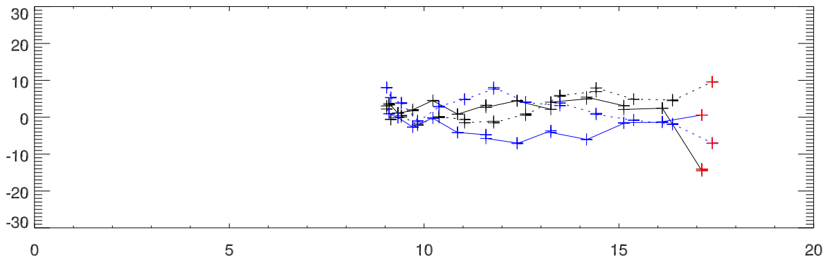
B2325+269 az,za error vs za
