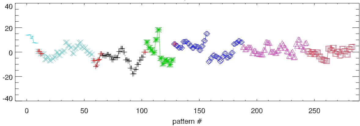
Az error vs pattern index
