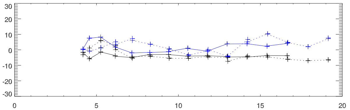
B0758+143 az,za error vs za
