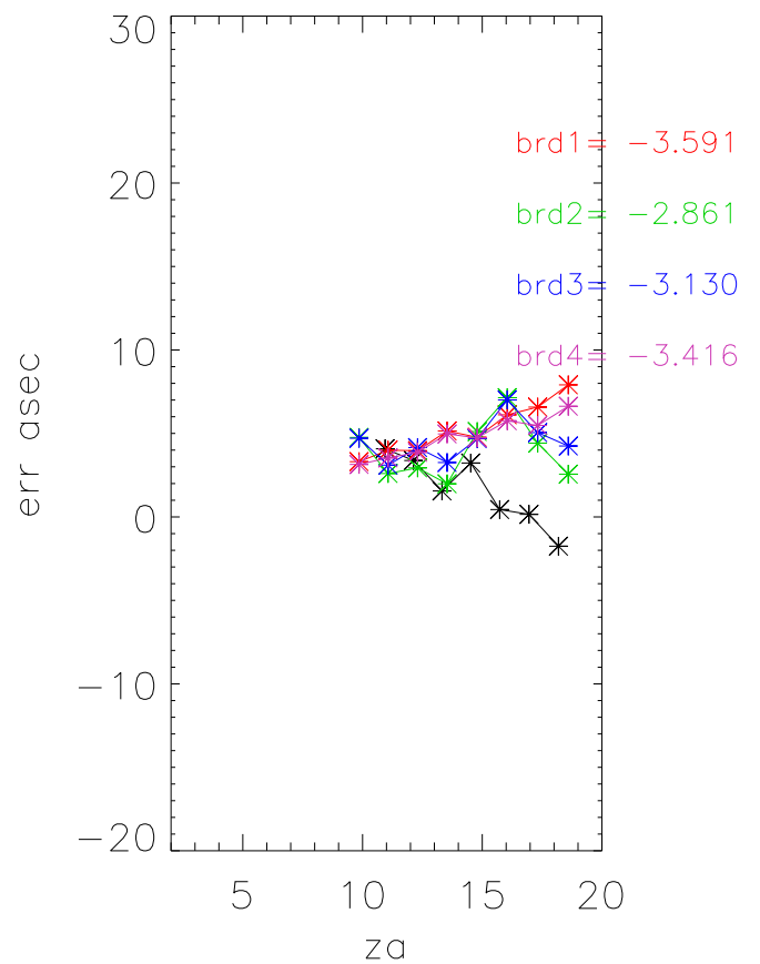
za Errors lbw J0141+138
