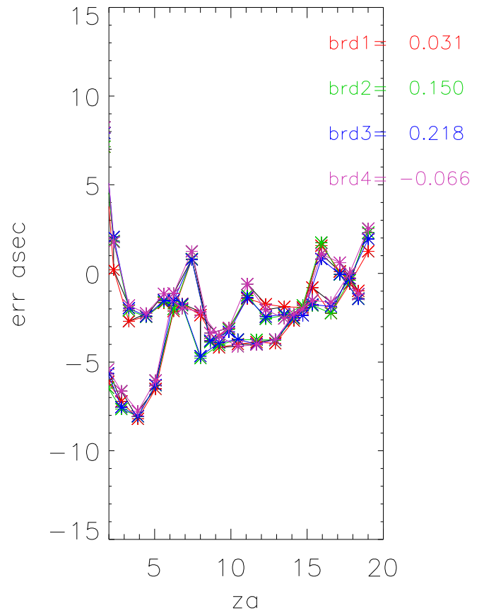
za Errors cb B0518+165
