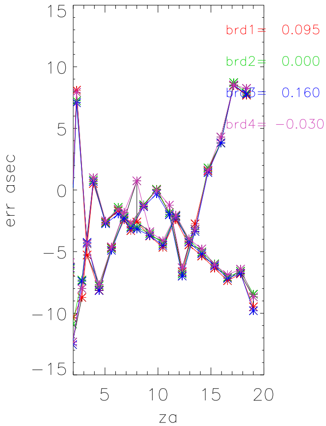
az Errors cb B0518+165
