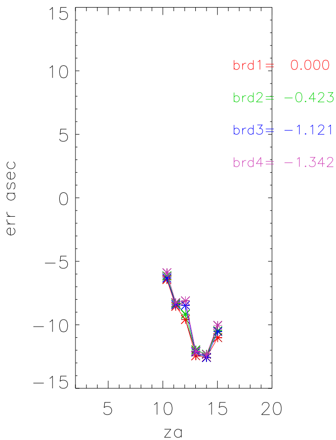
az Errors cb J0745+101
