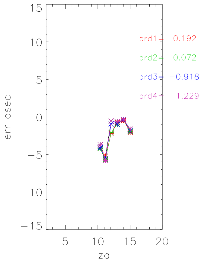
za Errors cb J0745+101
