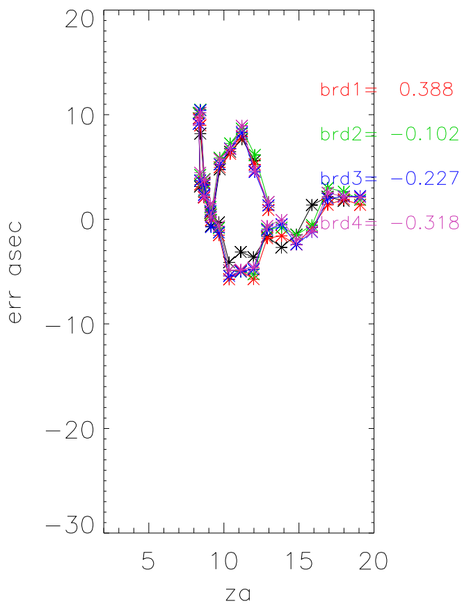
az Errors sbw B1607+268
