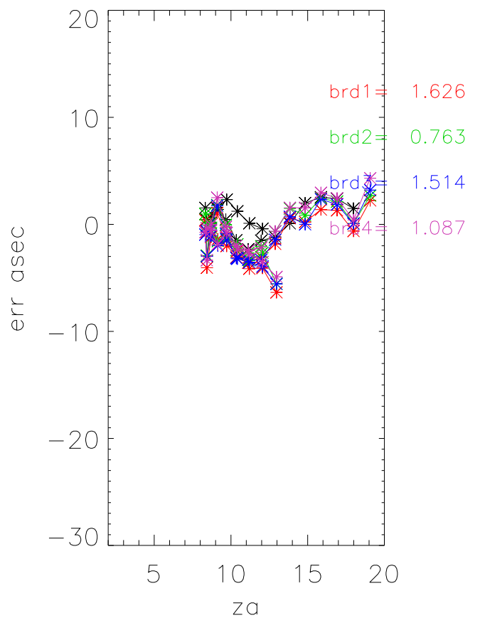
za Errors sbw B1607+268
