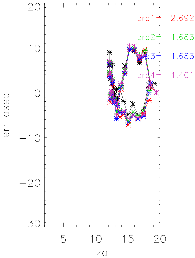
az Errors sbw B1328+307
