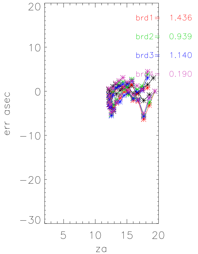
za Errors sbw B1328+307
