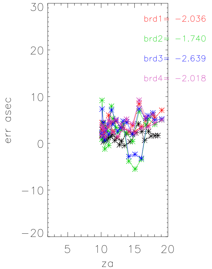
za Errors lbw B0949+287
