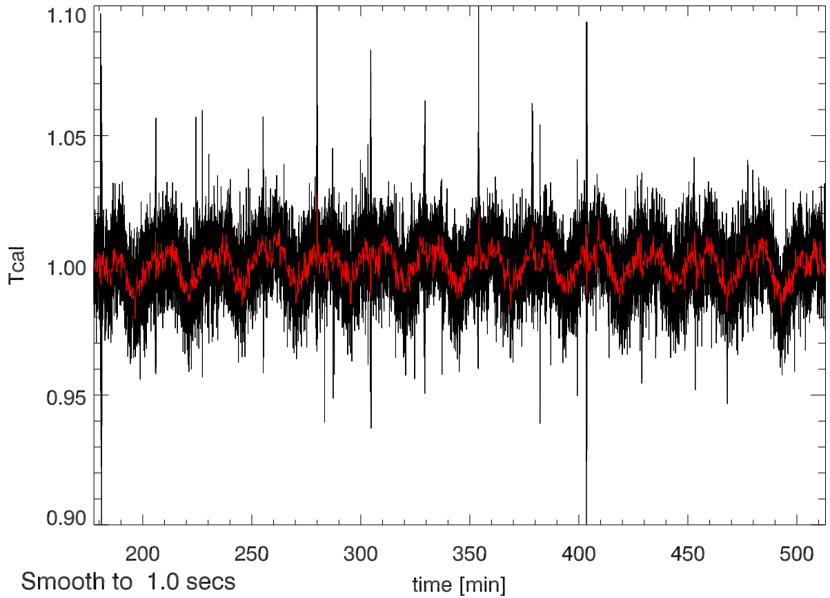
27jan13 calOn - calOff Beam2A SigA: 0.020
