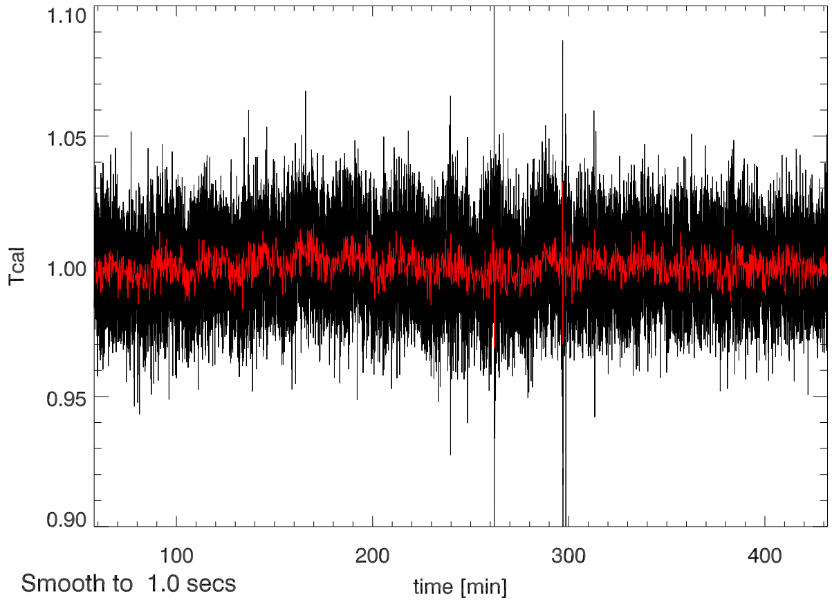
05jul11 calOn - calOff Beam2A SigA: 0.027
