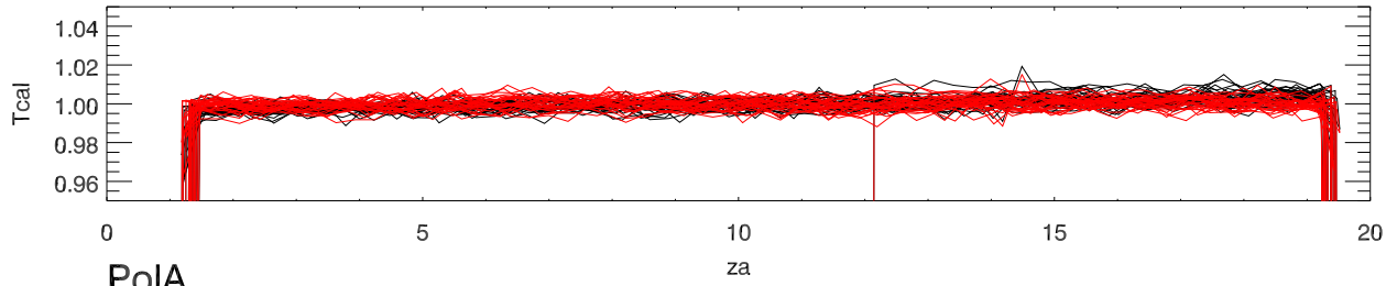
14jul11 a2130 alfaCalDeflection vs za beam0
