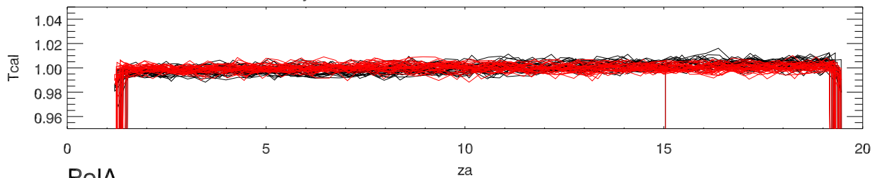
09jul11 a2130 alfaCalDeflection vs za beam0
