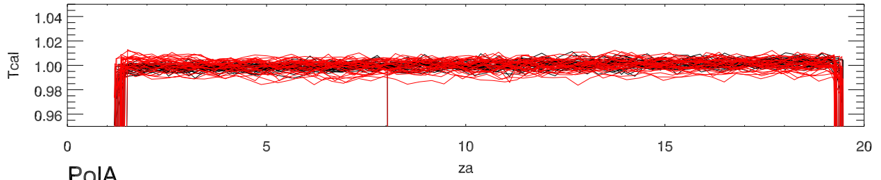
05jun11 a2130 alfaCalDeflection vs za beam0
