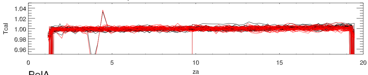
01jul11 a2130 alfaCalDeflection vs za beam0
