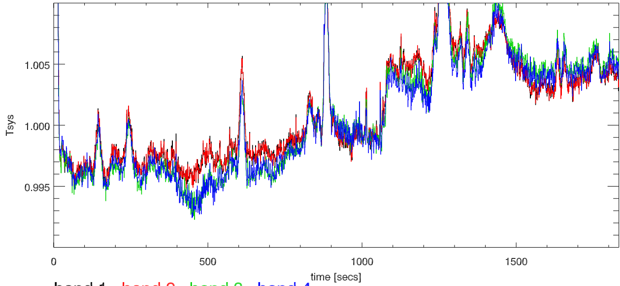
polB
