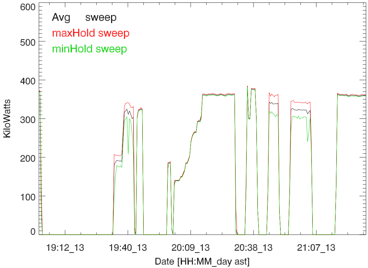
TxPwrTot. 13mar17:T3156. Paul Bernhardt 5 MHz
