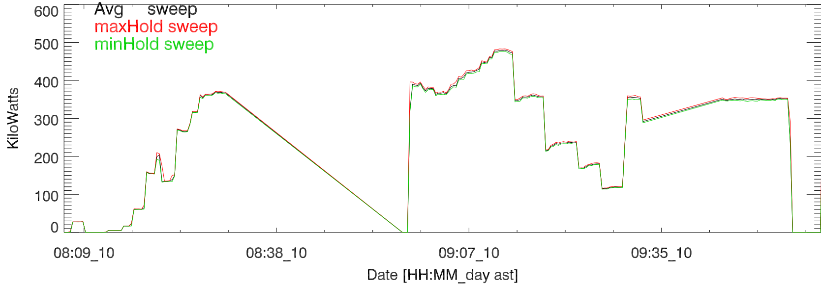
TxPwrTot. 10jun19:H3195 vladimir exp10.01 5 MHz
