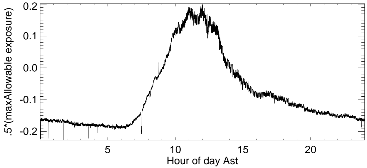
Rfmonitor data:091001
