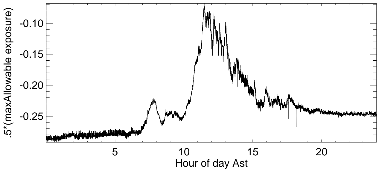
Rfmonitor data:091101
