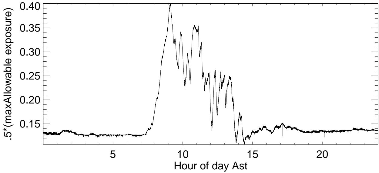
Rfmonitor data:090301
