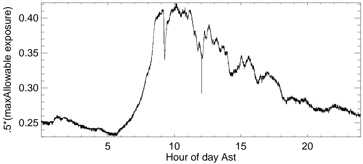
Rfmonitor data:090701
