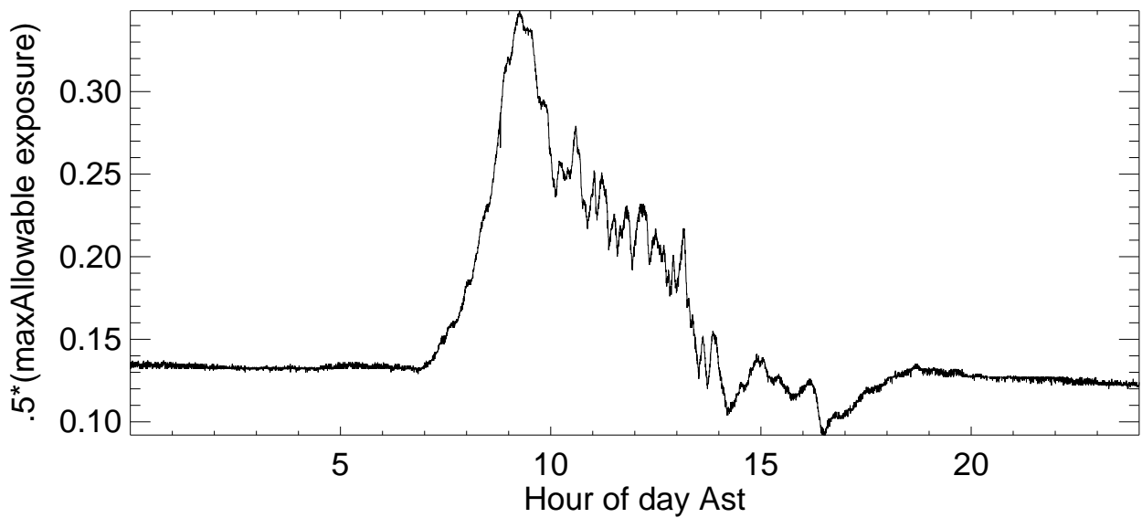
Rfmonitor data:090301
