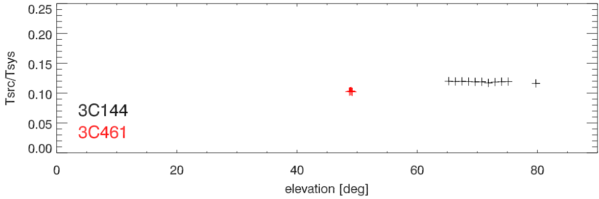
05-06may22 xband crosses. Tsrc/Tsys vs el CFR:8223.0MHz
