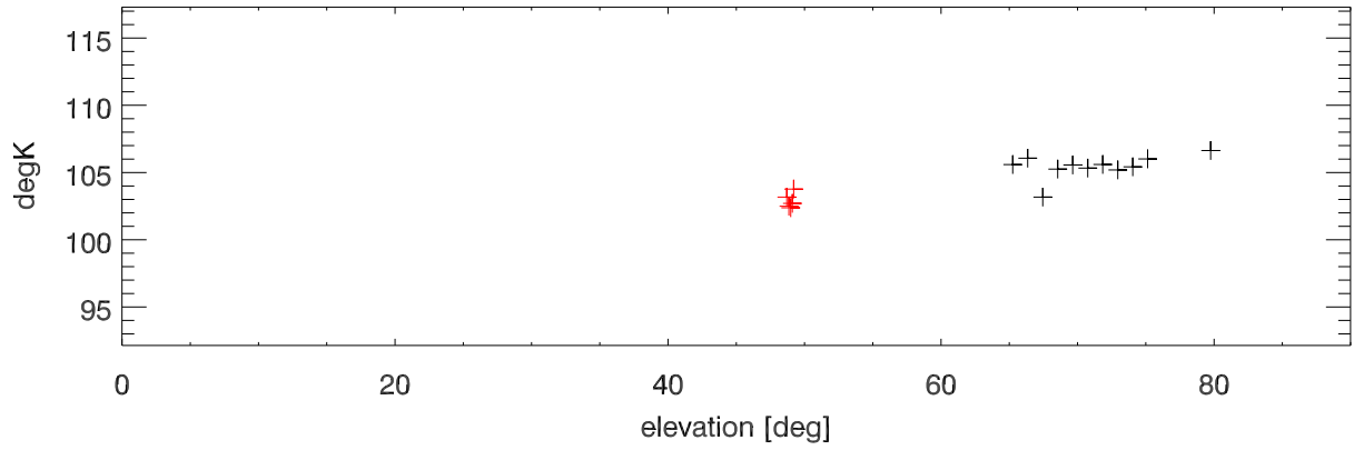
Tsys vs el
