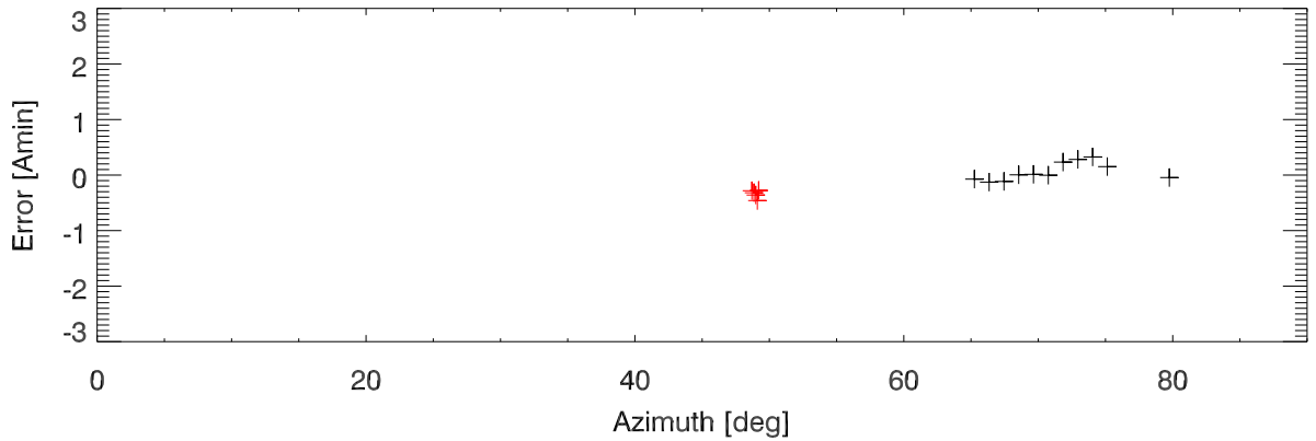
EI Pointing error vs el
