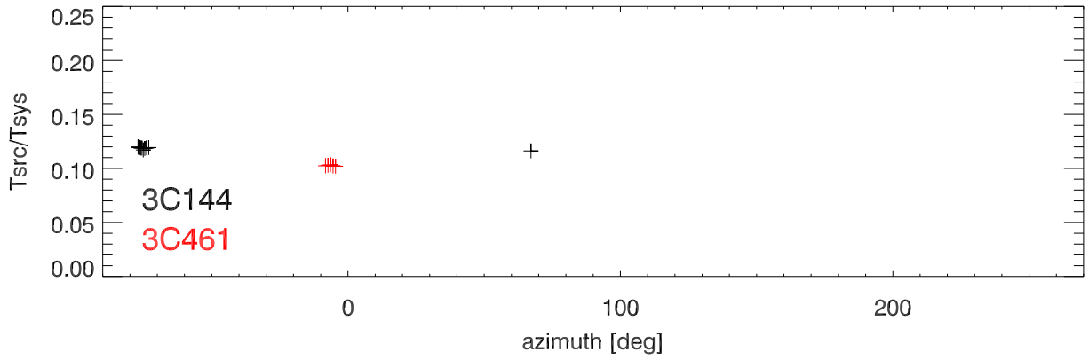
05-06may22 xband crosses. Tsrc/Tsys vs az CFR:8223.0MHz
