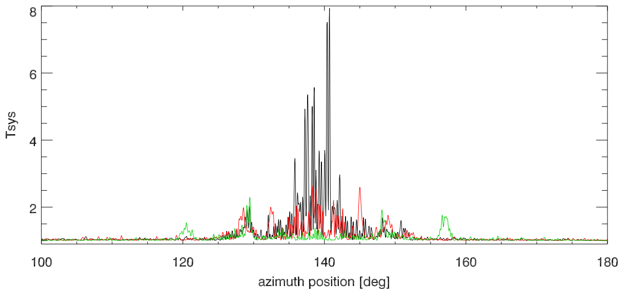
totPwr rfi vs az. rfi=8319.5 to 8348.7 MHz
