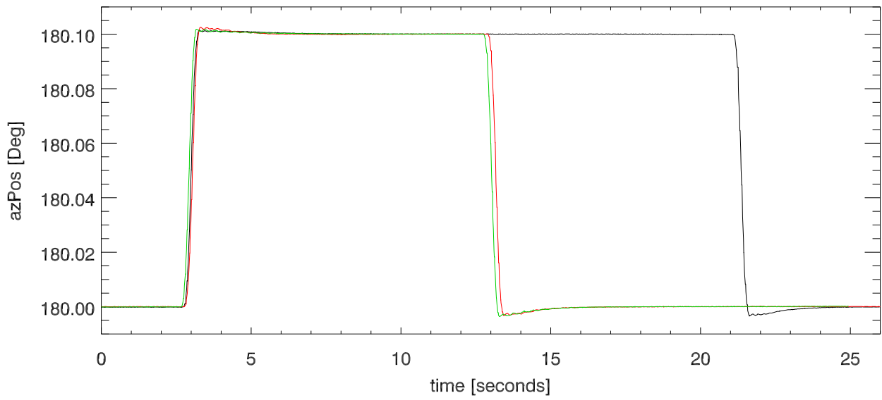
Az position vs Tm. AzStepSize=0.10 Deg
