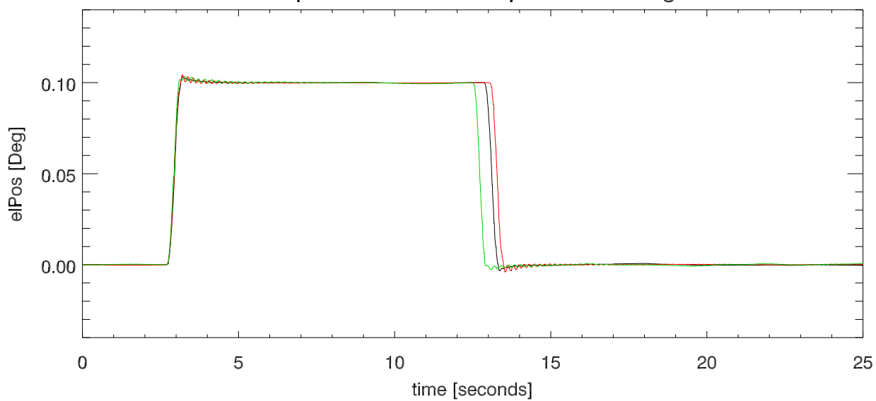
EI position vs Tm. EIStepSize=0.10 Deg
