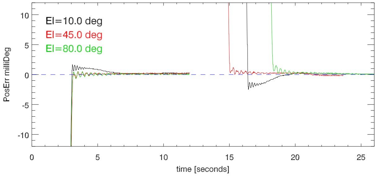
24jan11. Az step settling Error vs Tm. AzStepSize=0.02 Deg
