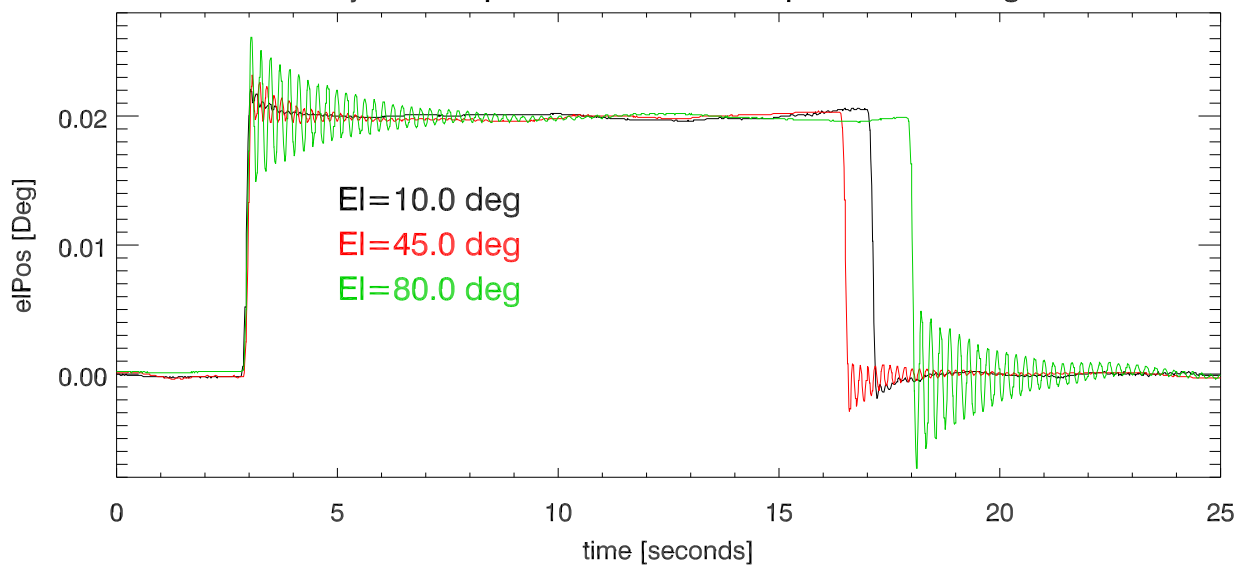
24jan11. EI position vs Tm. EIStepSize=0.02 Deg
