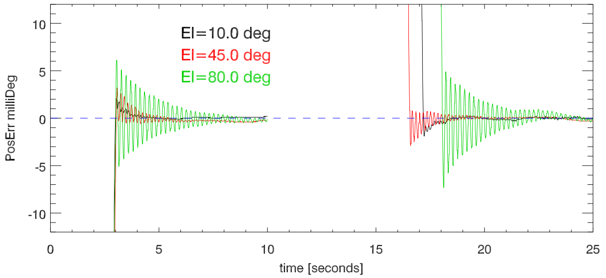
24jan11. EI step settling Error vs Tm. EIStepSize=0.02 Deg
