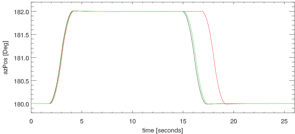
Az position vs Tm. AzStepSize=2.00 Deg
