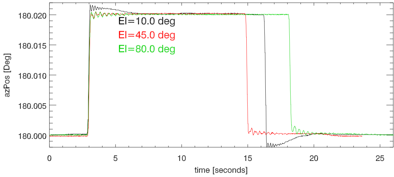
24jan11. Az position vs Tm. AzStepSize=0.02 Deg
